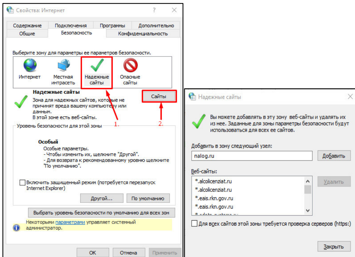
Рисунок 10 Надежные сайты
