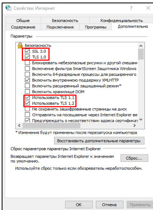
Рисунок 13 Дополнительно
