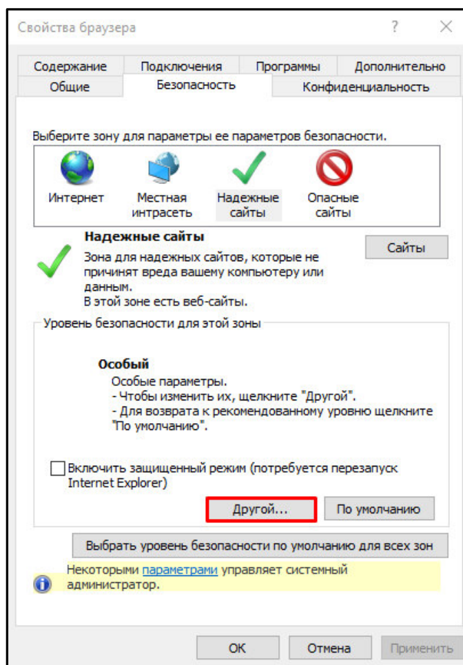
Рисунок 11 Свойства браузера
