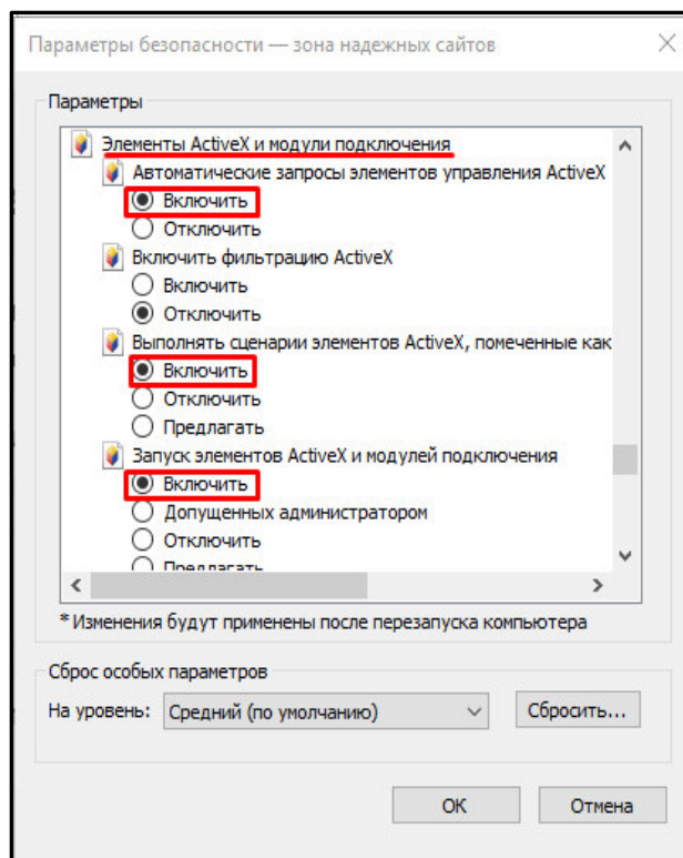
Рисунок 12 Параметры безопасности
